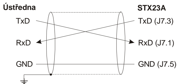
Obr. 7 – Propojení RS232
