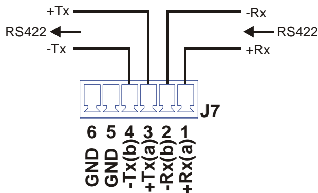
Obr. 10 - Propojení RS422
