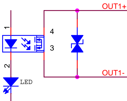
Obr. 2 - Schéma zapojení výstupního obvodu
