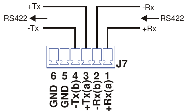
Obr. 11 - Propojení RS422
