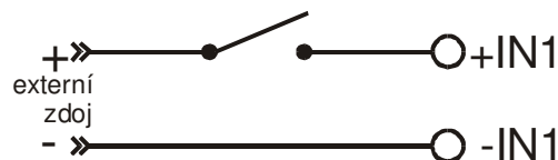
Obr. 7 - příklad zapojení vstupu
